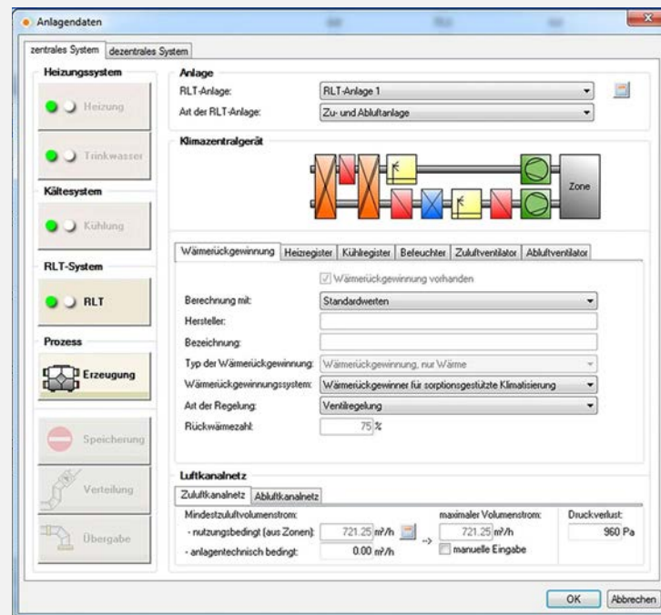
Abb. 22 Dialog zur Datenbearbeitung des Wärme-/Kälte-Erzeugers nach DIN V 18599 für ein Nicht-Wohngebäude im Rahmen der Nachweis-Erstellung nach GEG.
