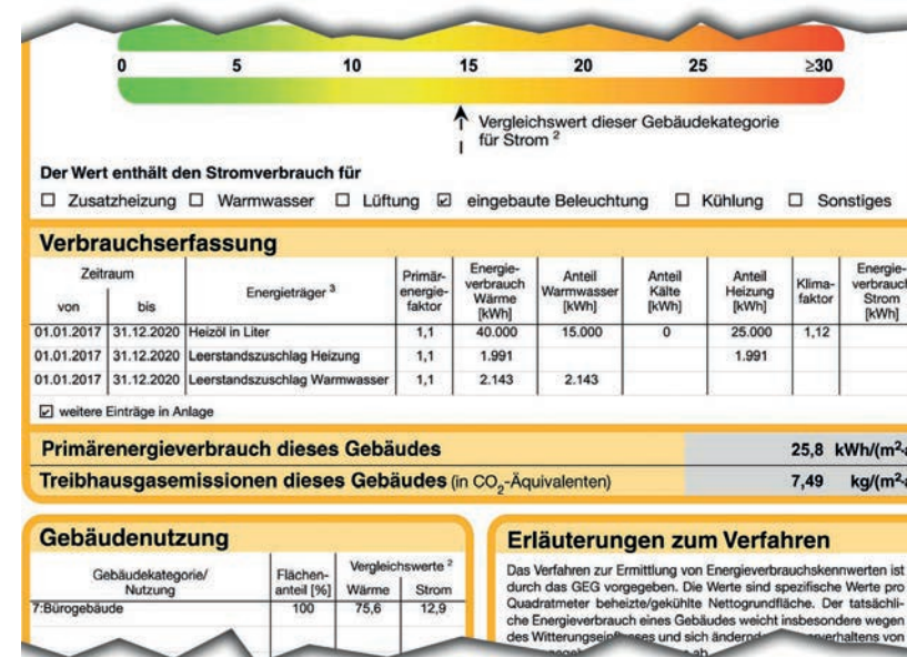
Abb. 25 Verbrauchsausweis (Auszug) nach GEG für ein Wohn- oder Nichtwohngebäude inkl. Nachweis der Treibhausgasemission (CO 2 -Äquivalent)
